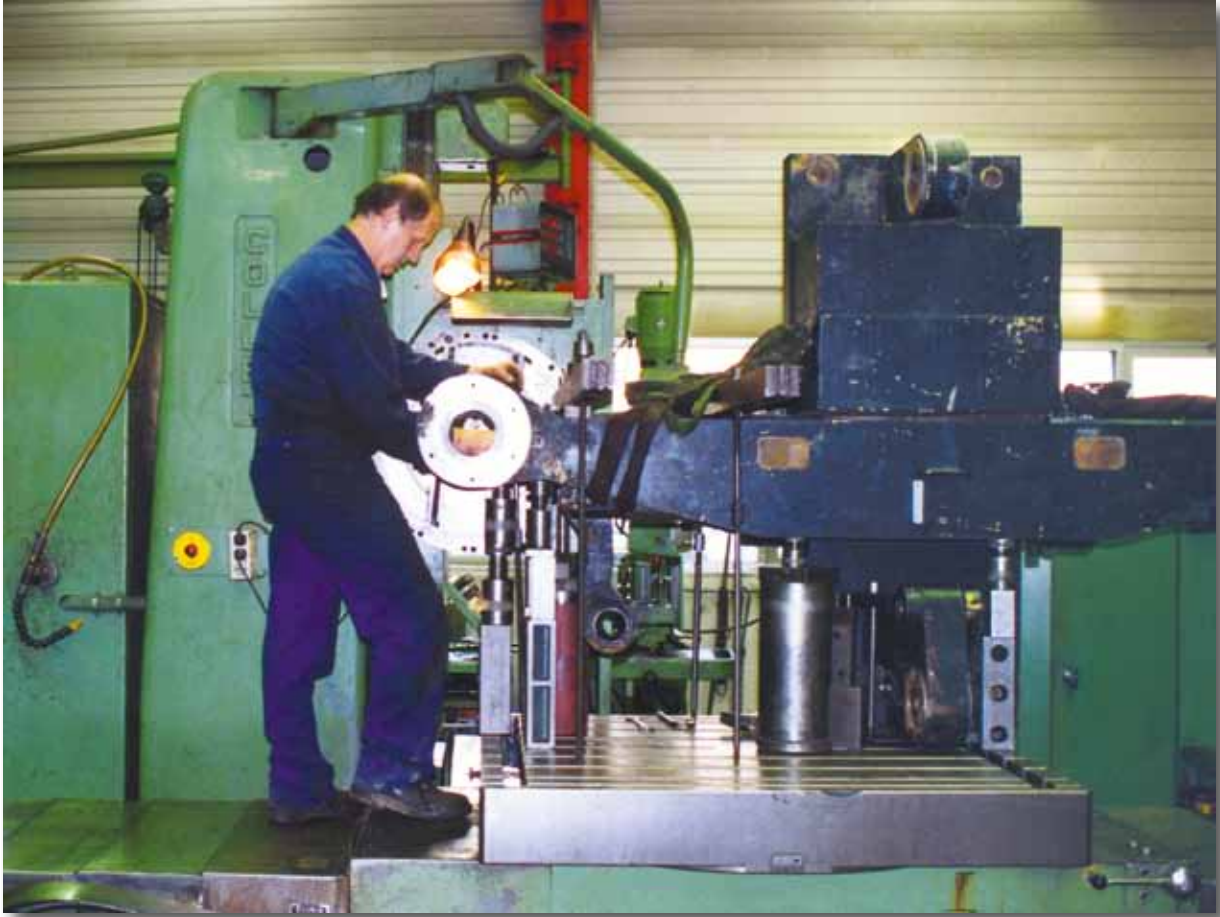
abgebrochenes Auge ansetzen und bohren
