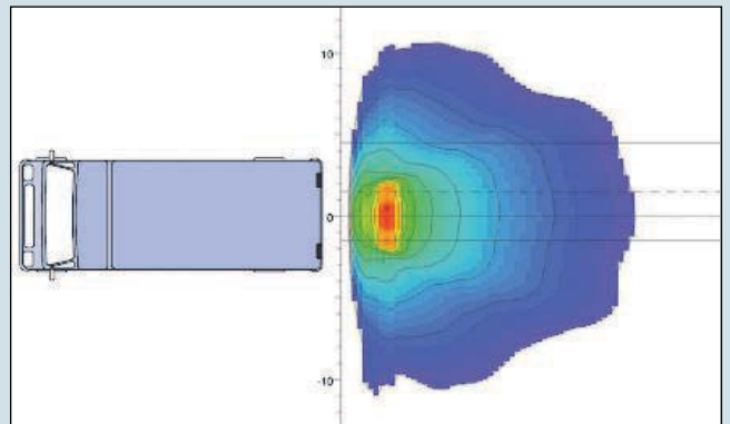
Abb. 2: Zwei zusätzliche Rückfahrscheinwerfer am Heck.
