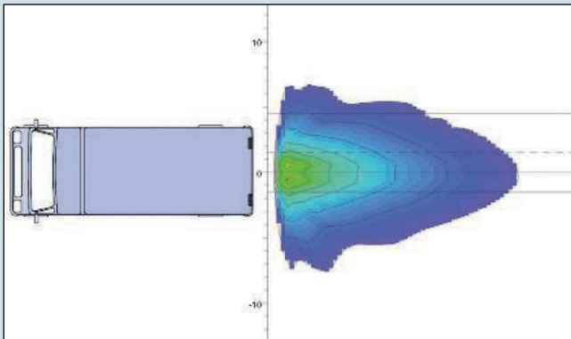
Abb. 1: Zwei Standard -Rückfahrscheinwerfer, gesetzlich vorgeschrieben.
