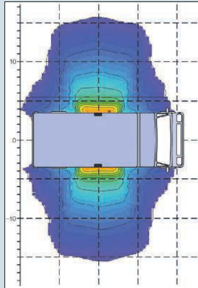
Abb. 4: Jeweils zusätzlich ein seitlicher Rückfahrscheinwerfer.
