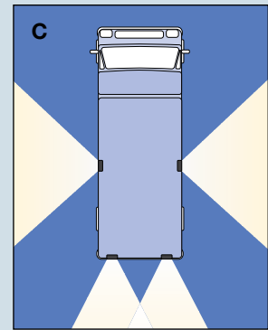
Variante C: Zwei zusätzliche Rückfahrscheinwerfer am Heck plus jeweils ein zusätzlicher Rückfahrscheinwerfer pro Seite
