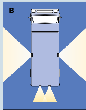
Variante B: Jeweils ein zusätzlicher Rückfahrscheinwerfer pro Seite
