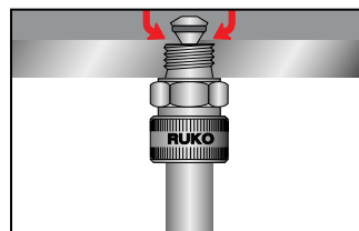
Ablasskupplung aufschrauben
