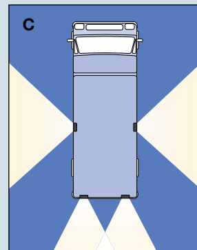
Variante C: Zwei zusätzliche Rückfahr- scheinwerfer am Heck plus jeweils ein zusätzlicher Rück- fahrcheinwerfer pro Seite
