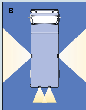
Variante B: Jeweils ein zusätzlicher Rückfahrcheinwerfer pro Seite
