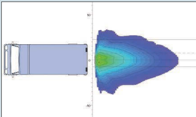
Abb. 1: Zwei Standard -Rückfahrcheinwerfer, gesetzlich vorgeschrieben.
